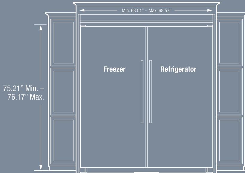
79" TRMKTSS2FL79– Flat
